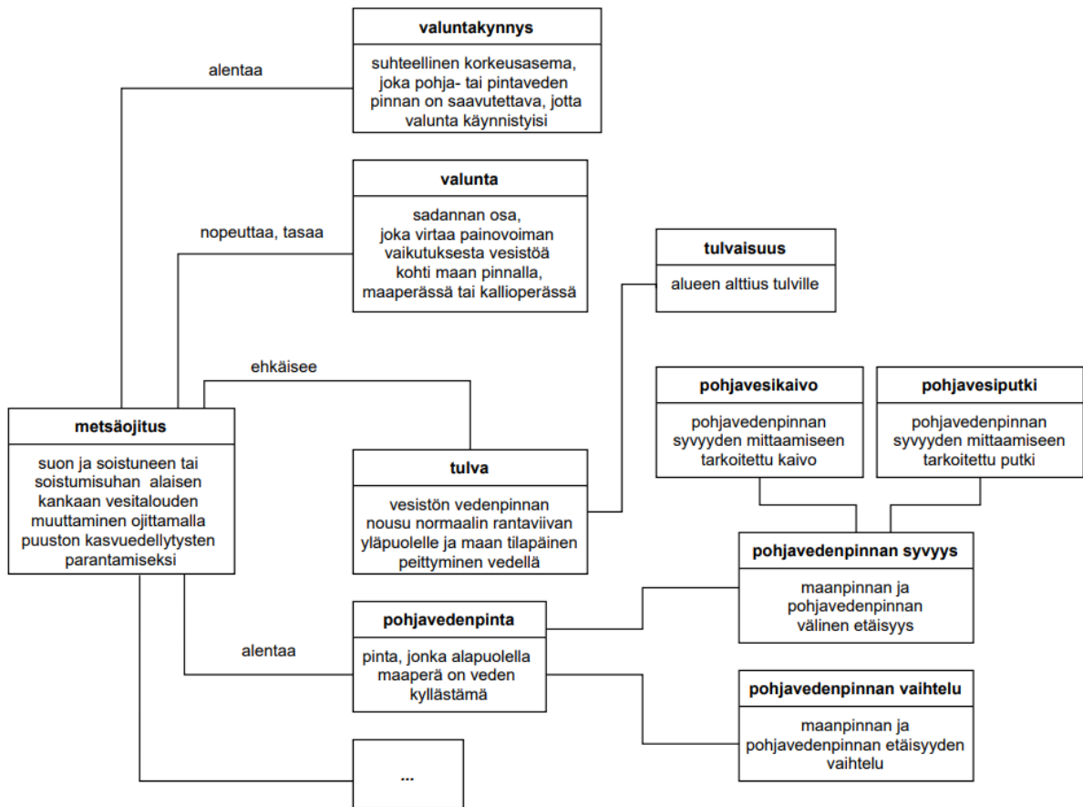
Käsitekaavio 12. Metsäojituksen hydrologiset vaikutukset ojitusalueilla.
