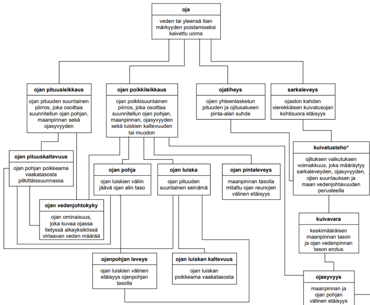
Käsitekaavio 10. Ojan ominaisuudet ja tunnukset.
