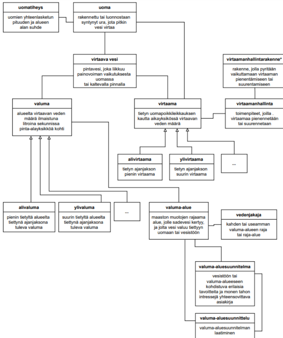
Käsitekaavio 3. Virtaavaan veteen liittyvät käsitteet.
