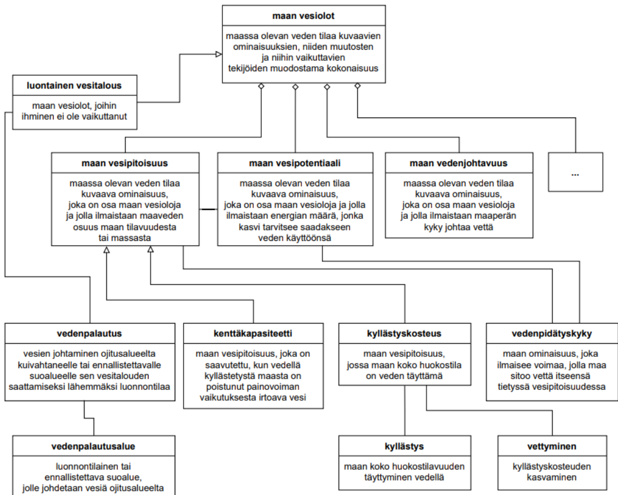
Käsitekaavio 15. Maan vesiolot.
