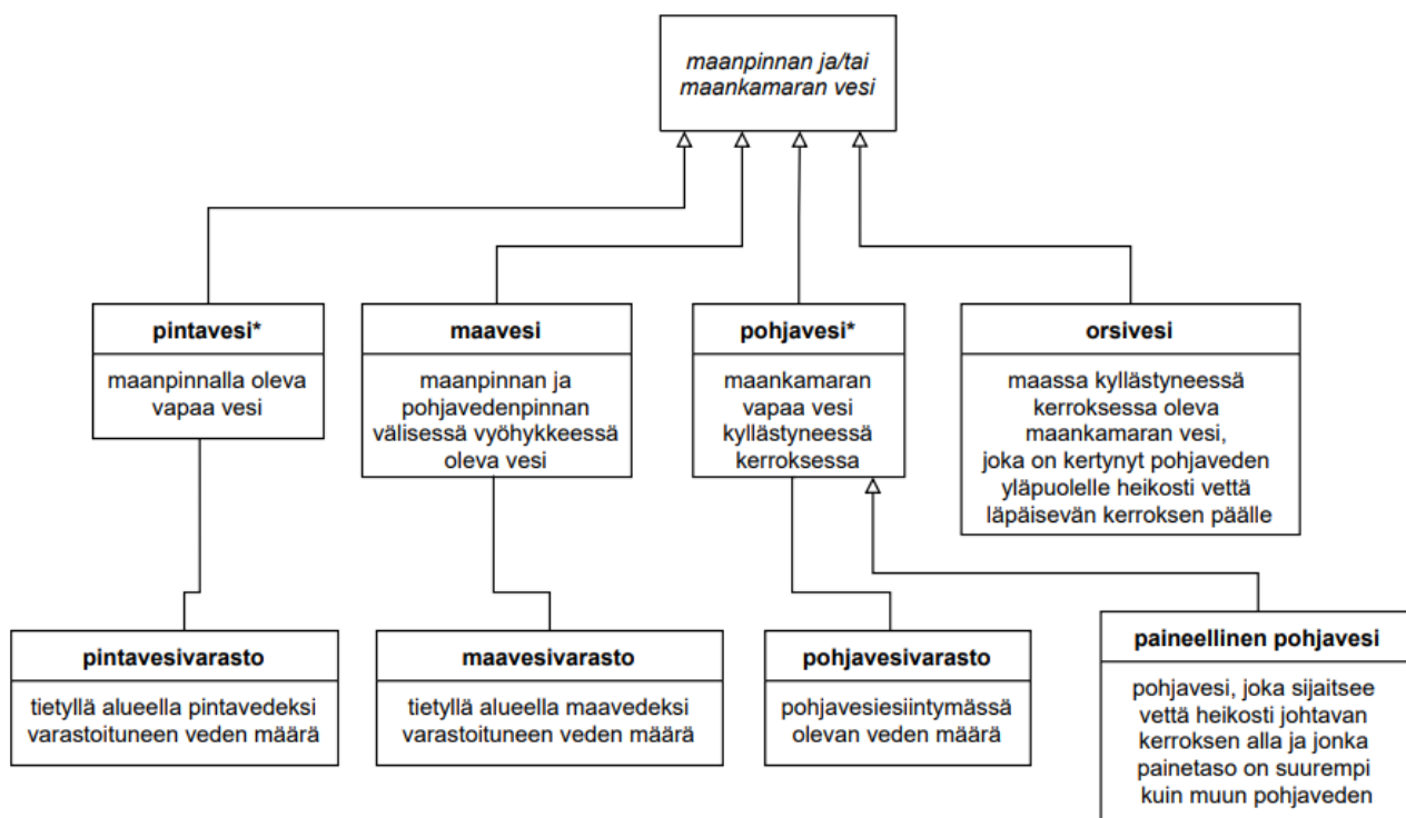
Käsitekaavio 1. Vesi ja vesivarastot
