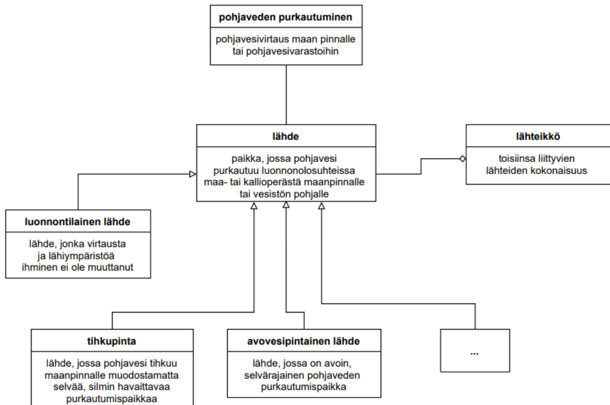
Käsitekaavio 5. Pohjaveden purkautuminen.
