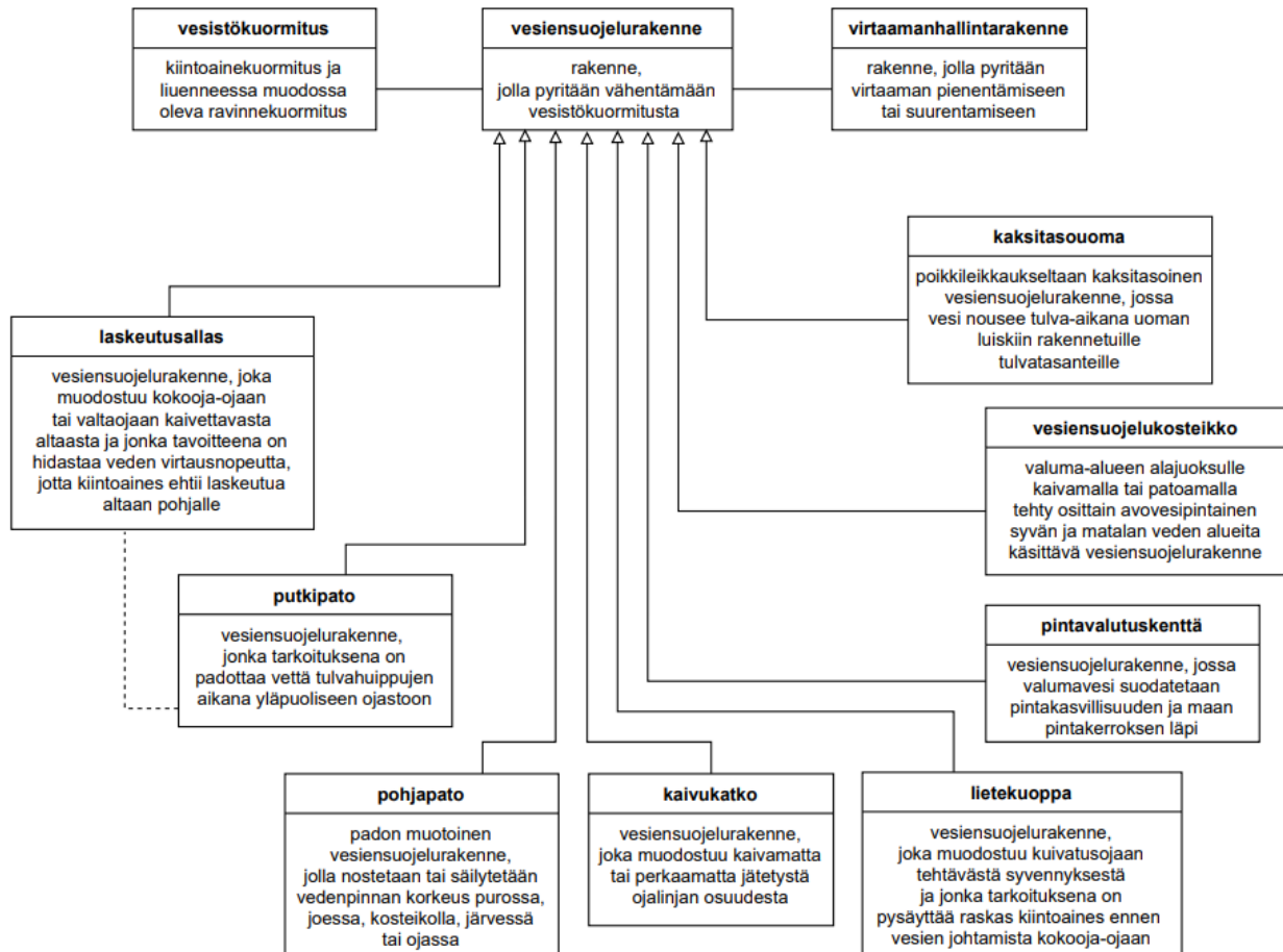
Käsitekaavio 13. Metsäojituksessa käytettävät vesiensuojelurakenteet.
